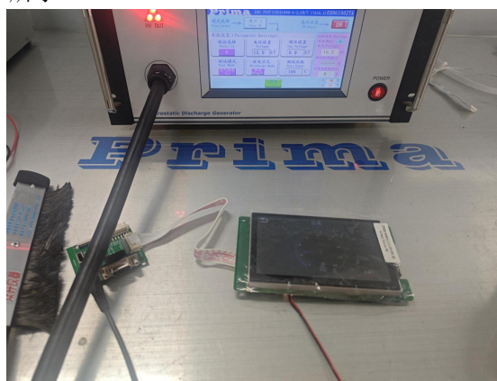
图 4-2 ESD 测试图
