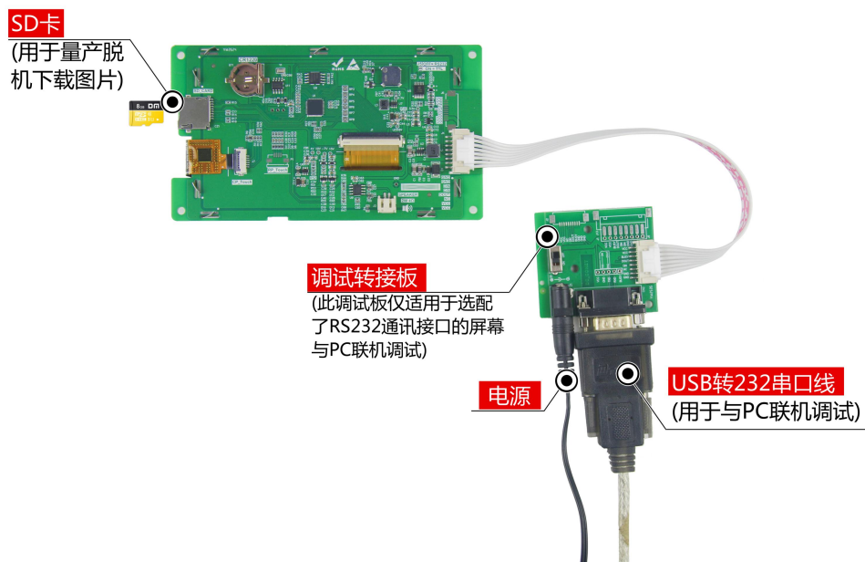
图 1-5 调试工具图
