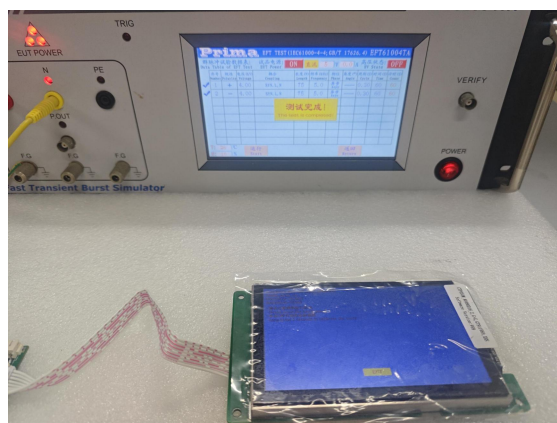
图 4-3 EFT 测试图
